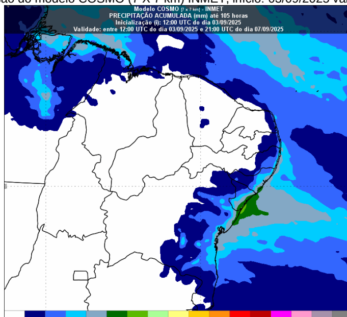
Figura 1 - Previsão do modelo COSMO (7 X 7 km) INMET, início: 03/09/2025 validade: 07/09/2025
