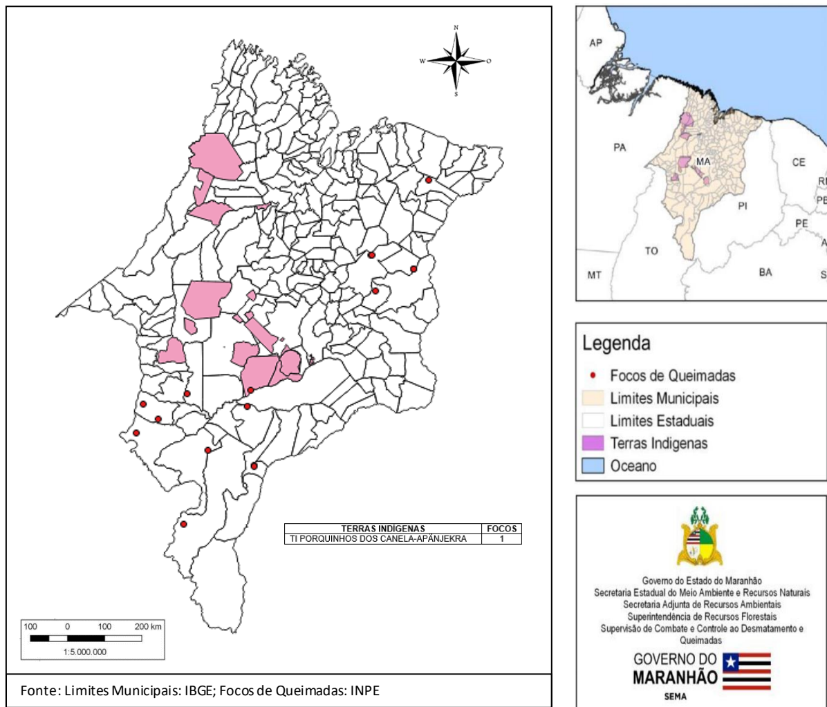
Figura 04: Focos de queimadas entre o dia 16 a 31 de março de 2022. Fonte: SEMA/2022; INPE/2022.
