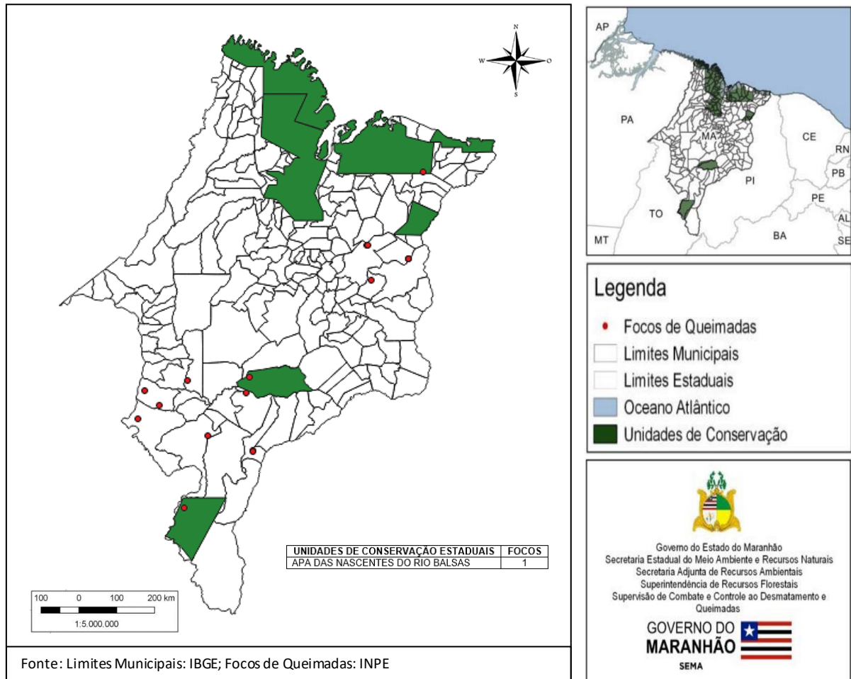
Figura 03: Focos de queimadas entre o dia 16 a 31 de março de 2022. Fonte: SEMA/2022; INPE/2022.
