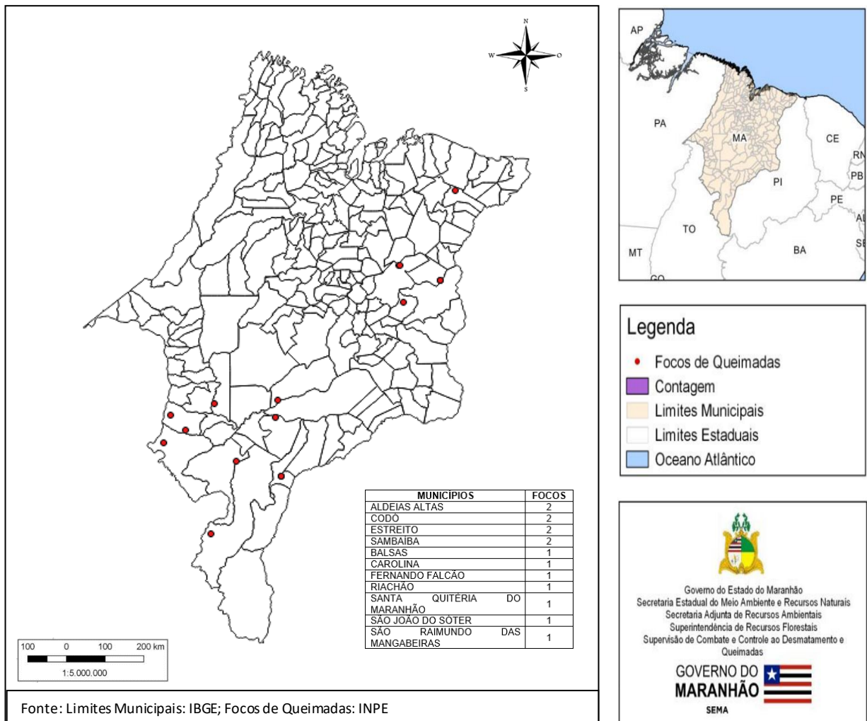
Figura 01: Focos de queimadas entre o dia 16 a 31 de março de 2022. Fonte: SEMA/2022; INPE/2022.
