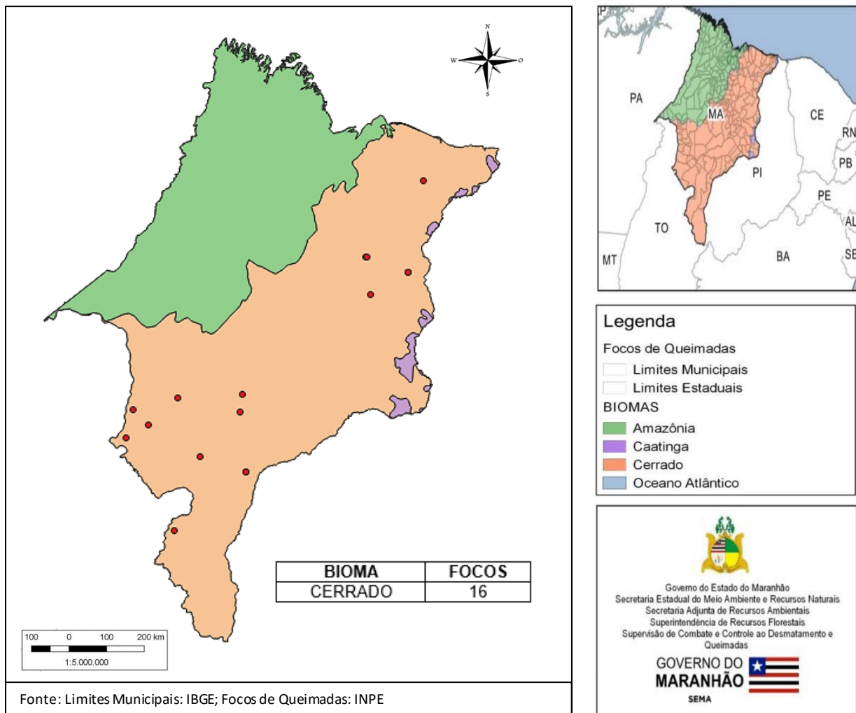
Figura 02: Focos de queimadas entre o dia 16 a 31 de março de 2022. Fonte: SEMA/2022; INPE/2022.
