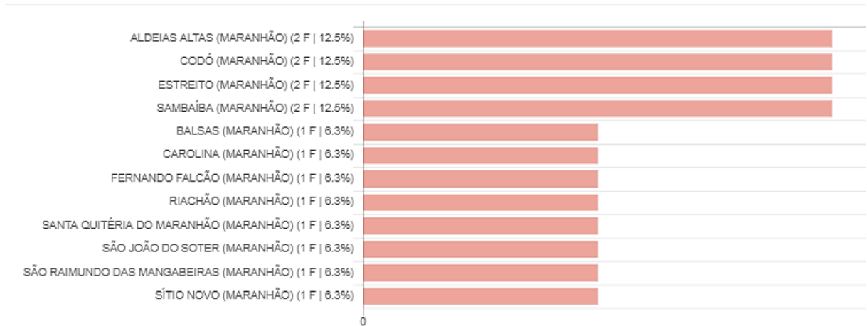
Figura 05: Gráfico com números de focos de queimadas entre o dia 16 a 31 de março de 2022. Fonte: INPE/2022.
